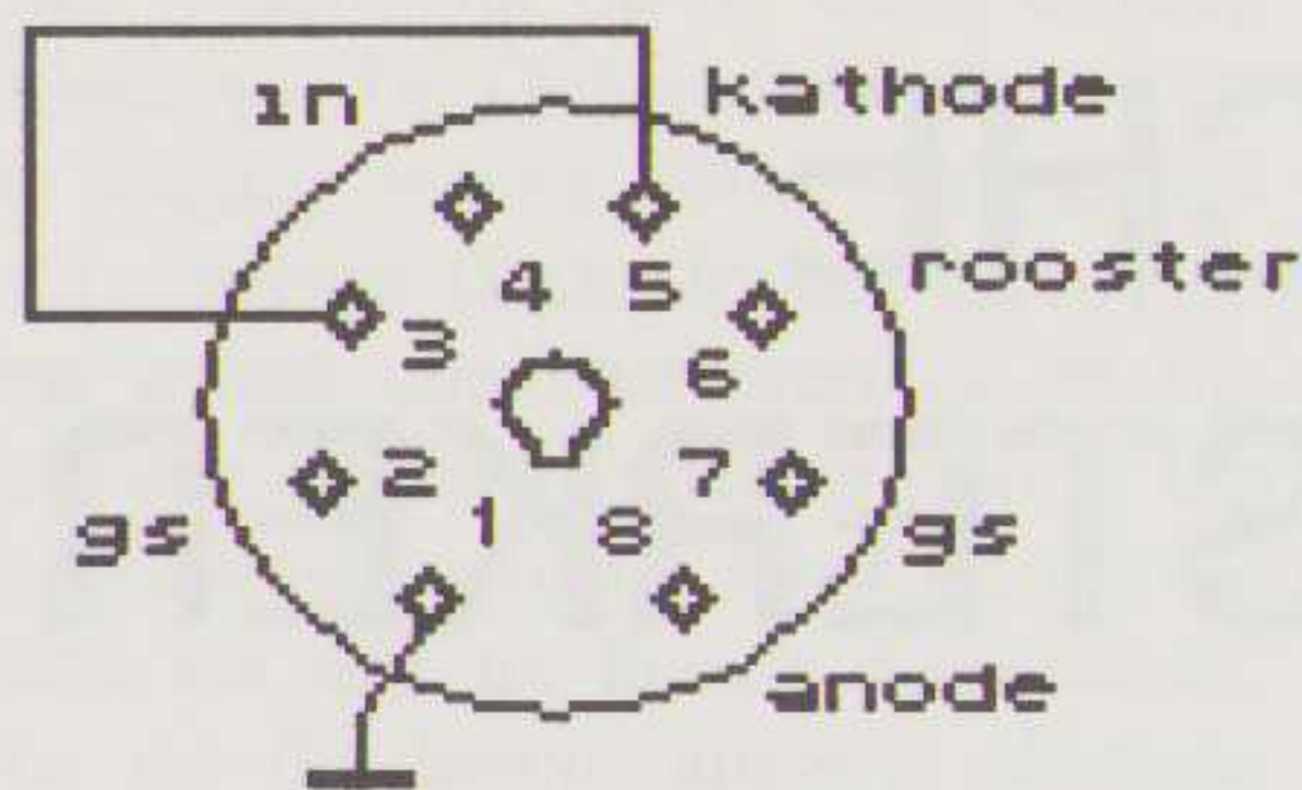
6SJ7
